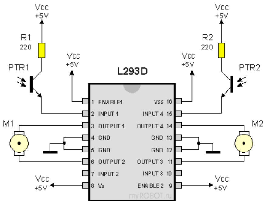
Схема робота с двумя фототранзистрами
